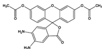
Struktur von DAF- 2 DA Structure of DAF-2 DA
