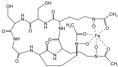
Strukturformel von Ferrichrysin (eisenhaltige Form) Structural formula of Ferrichrysin (ferric form)
